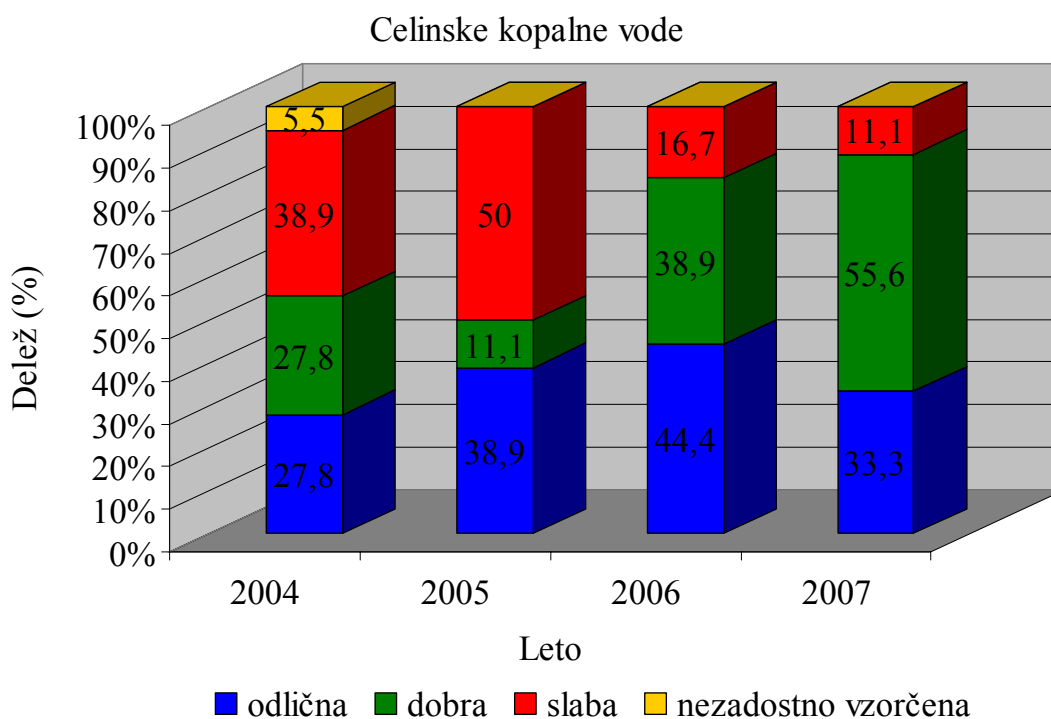
Slika 21: Skladnost celinskih kopalnih voda z zahtevami direktive
