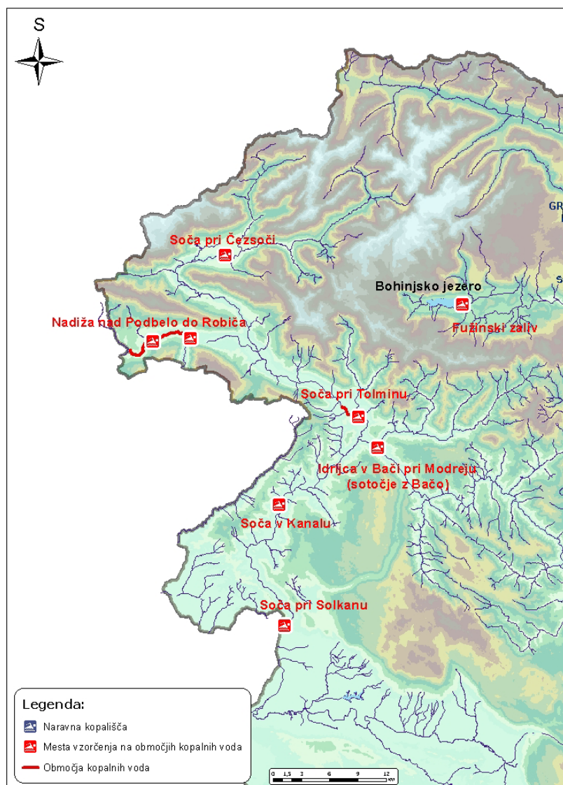
Slika 3: Kopalne vode na Goriškem in Gorenjskem
