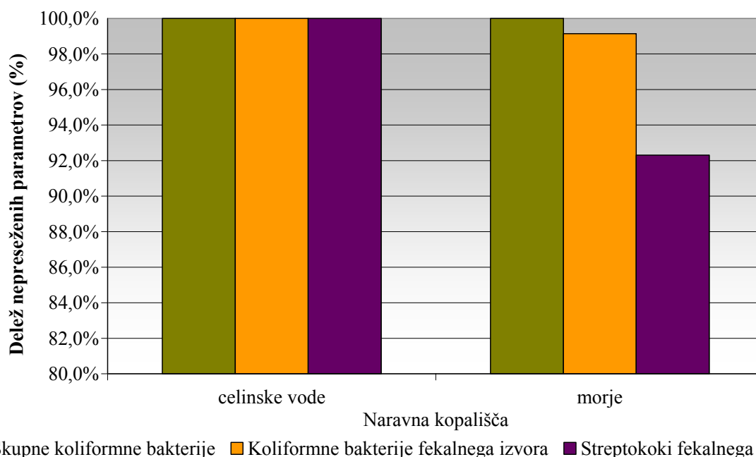
Slika 8: Delež skladnih mikrobioloških parametrov glede na mejne vrednosti po pravilniku, na naravnih kopališčih, v letu 2007
