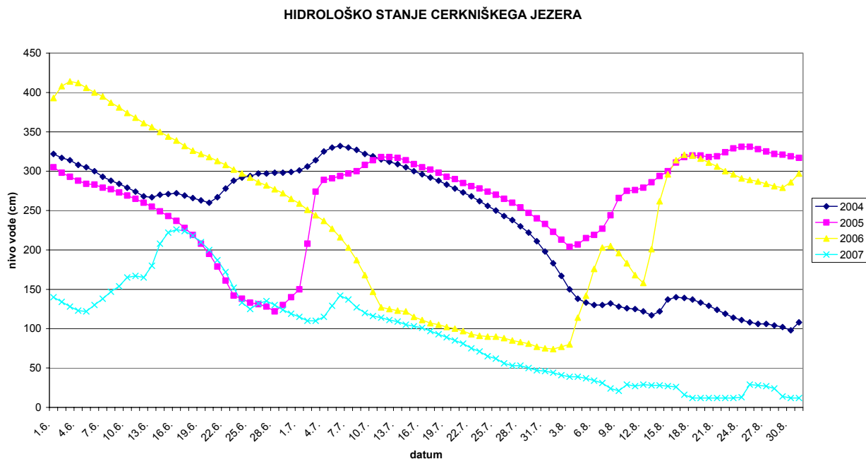
Slika 12: Srednji dnevni vodostaji na postaji Dolenje jezero na Cerknjskem jezeru v letih 2004-2006
